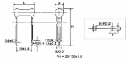
Radial type-TMOR
